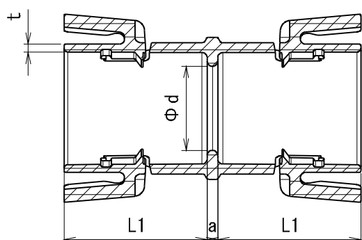
断面 A-A
